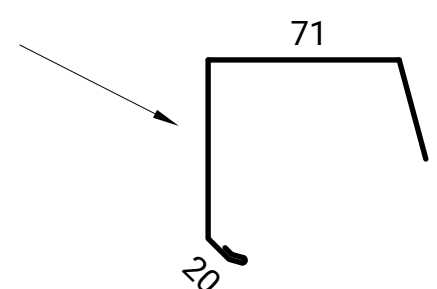
CORONACIÓN VUELO TROQUELADA AIS TAP/3G/5G
