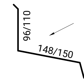
FALDÓN TRASERO TROQUELADO AIS TAP/3G/5G
