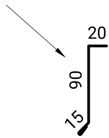
FRONTAL TROQUELADO AIS COPPO PLIEGUE EXTERIOR
