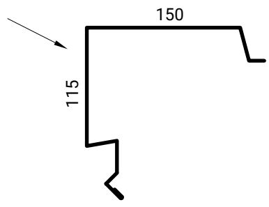
CORONACIÓN LATERAL AIS TAP/3G/5G
