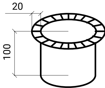
BOQUILLA BAJANTE CANALÓN GALVANIZADA
