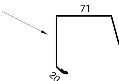
CORONACIÓN VUELO TROQUELADA AIS TAP/3G/5G
