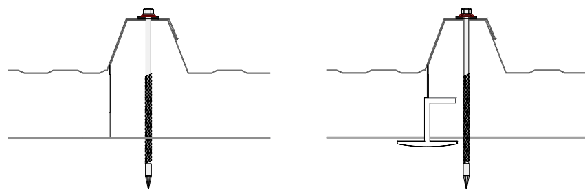
DETALLE DE UNIÓN
