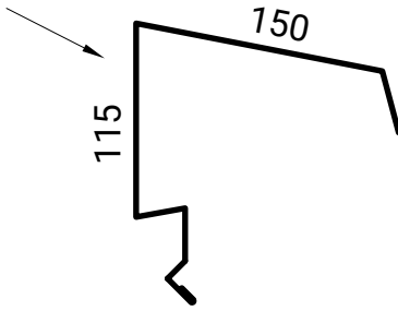
CORONACIÓN TRASERA TROQUELADA AIS TAP/3G/5G
