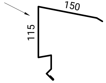
CORONACIÓN TRASERA SIN TROQUELAR
