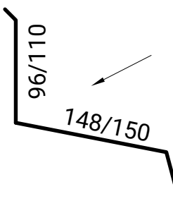
FALDÓN TRASERO TROQUELADO AIS TAP/3G/5G
