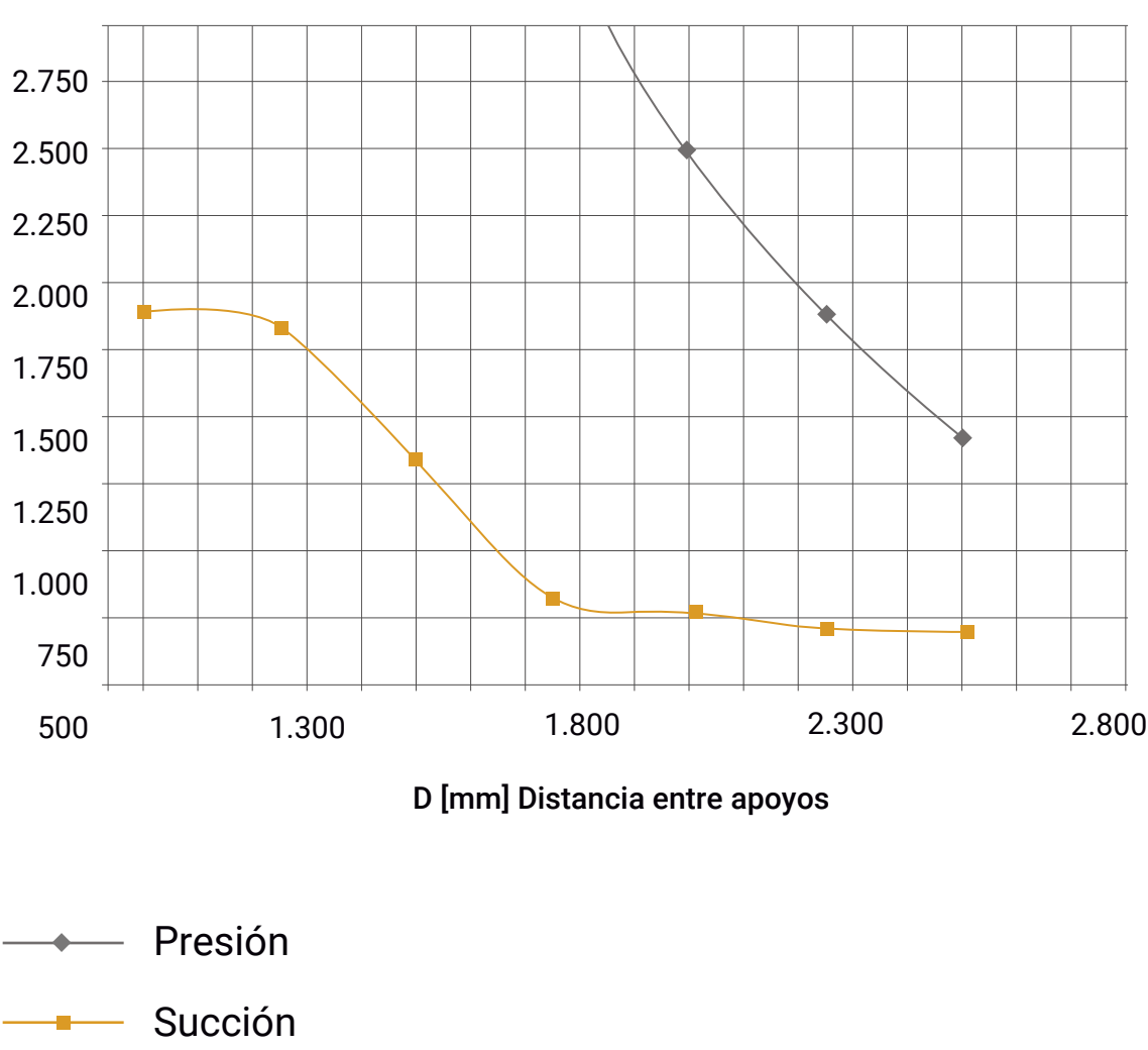
Propiedades estáticas (kg/m2)
