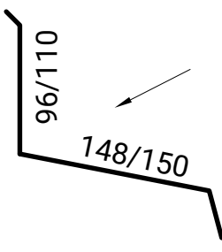
FALDÓN TRASERO TROQUELADO AIS TAP/3G/5G
