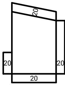
BOQUILLA BAJANTE CANALÓN GALVANIZADA
