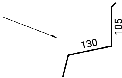
FALDÓN TRASERO TROQUELADO AIS COPPO
